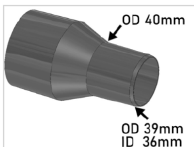
Stofvoeradapter - Afmetingen slangkoppelingen
